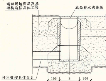
集水井侧排水管安装详图 (二)
