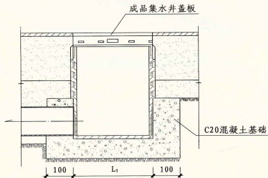
集水井侧排水管安装详图 (一)
