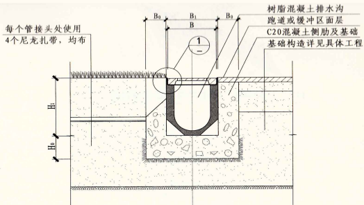
成品排水沟安装详图
